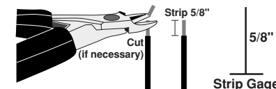
Strip Gage
