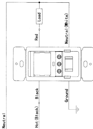
Wiring Diagram:
