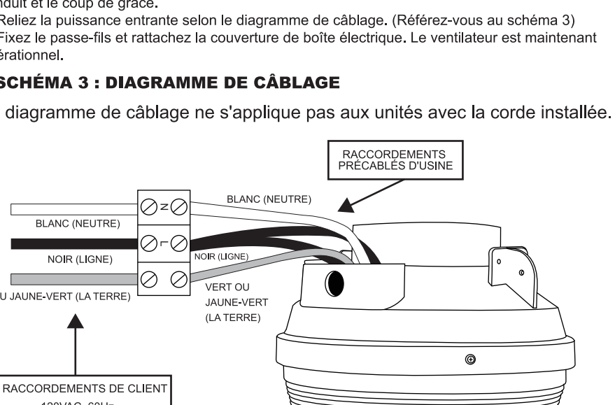
LE SCHEMA 3 : DIAGRAMME DE CÂBLAGE
