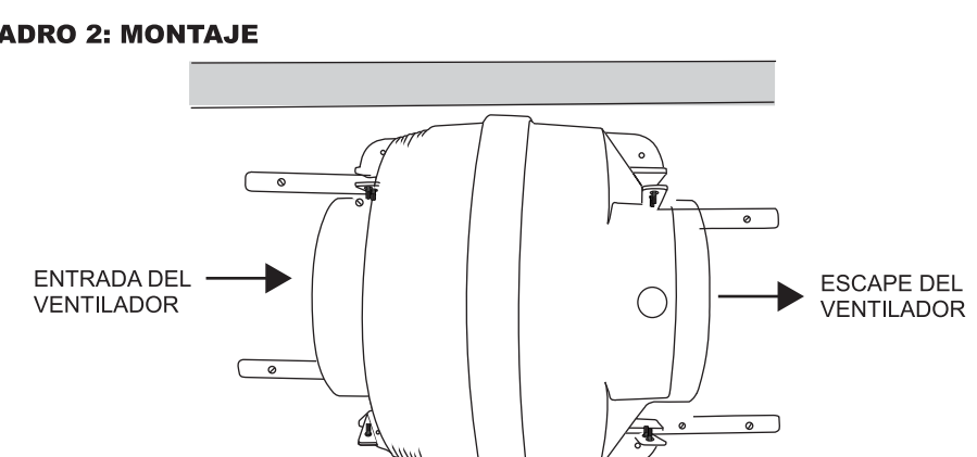
CUADRO 2: MONTAJE
