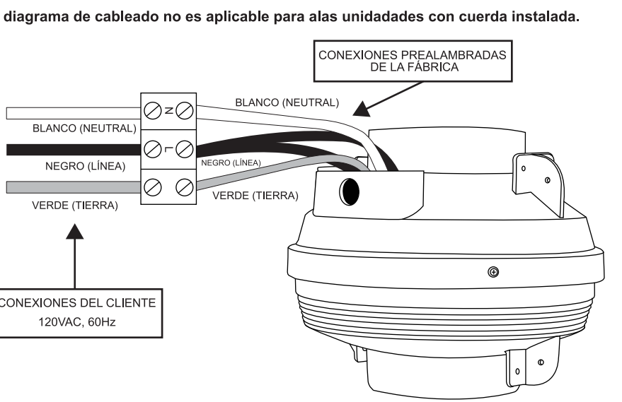
CUADRO 3: DIAGRAMA DE CABLEADO
