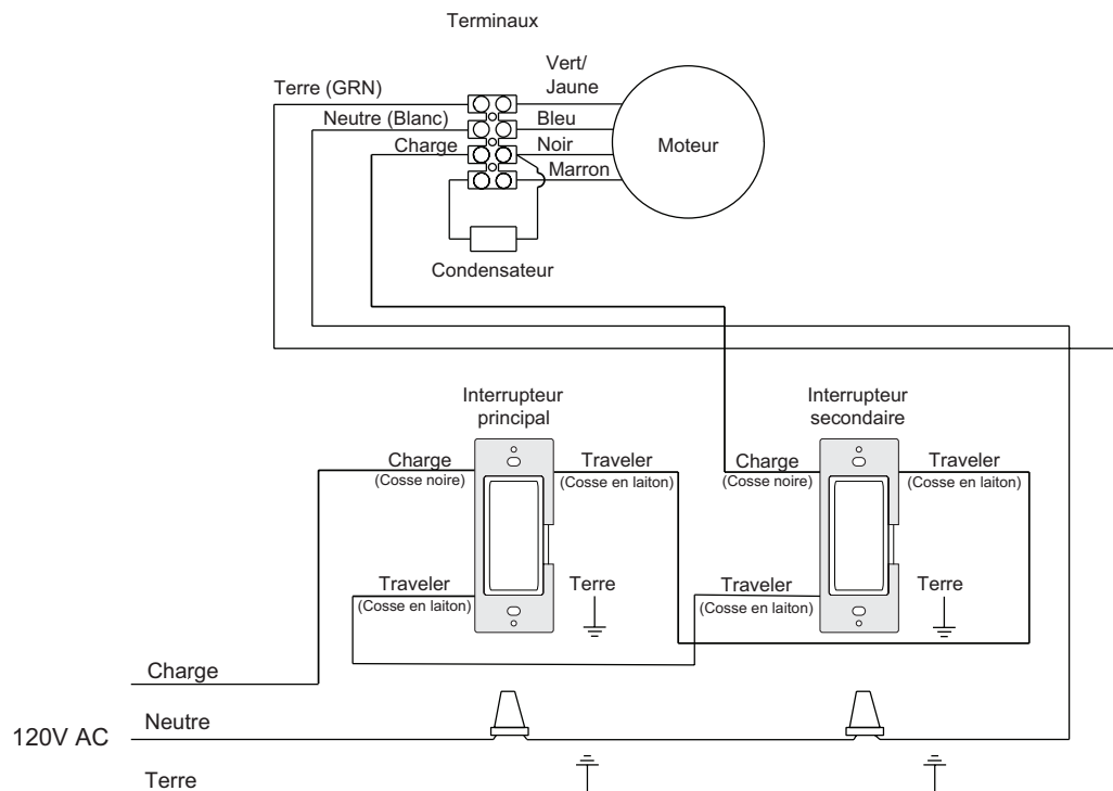
Deux interrupteurs d'éclairage pour deux emplacements (séries PB 270 et PB 370-2)
