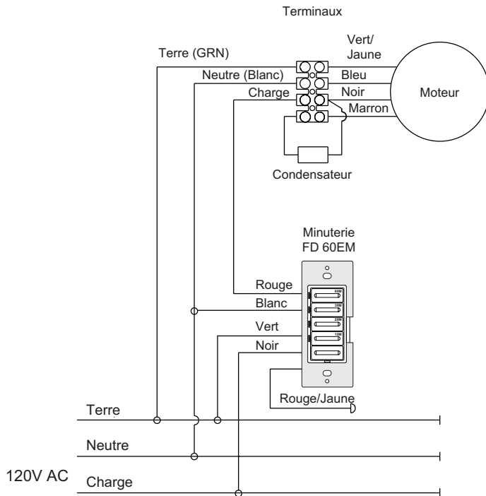
Minuterie FD 60EM pour Single (séries PB 110)
