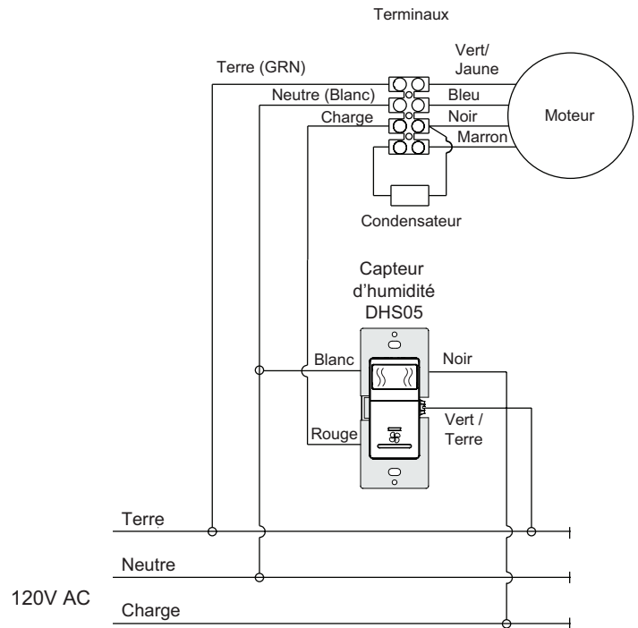
Capteur d'humidité DHS05 pour un emplacement unique (séries PB 110)
