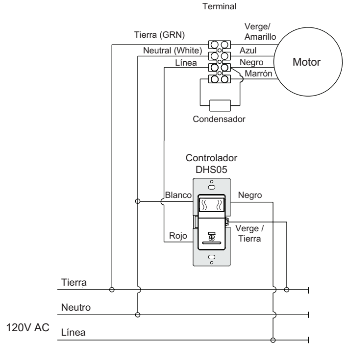
Sensor de humedad DHS05 para ubicación única (PB110)
