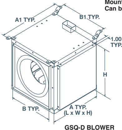
GSQ-D BLOWER
